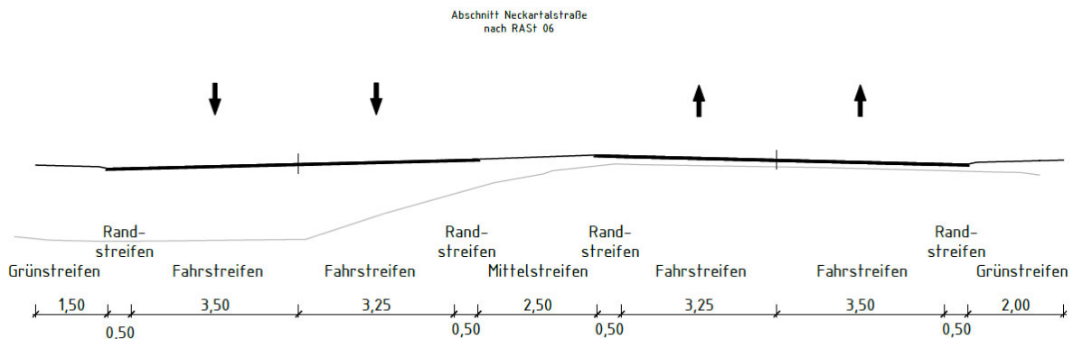
Abbildung 5: Regelquerschnitt Neckartalstraße
