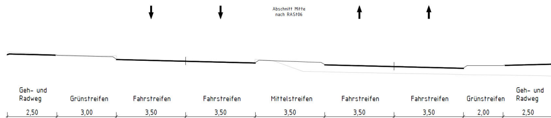
Abbildung 2: Regelquerschnitt Nordumfahrung Abschnitt Mitte
