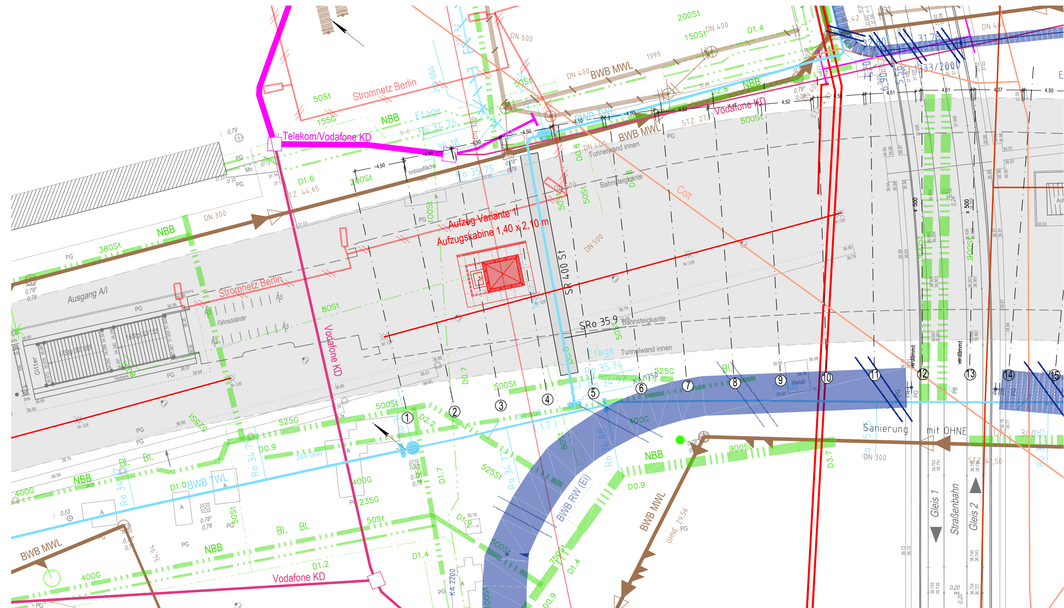
Grundriss Straßenebene und Standortvariante 1 (M 1:200)
