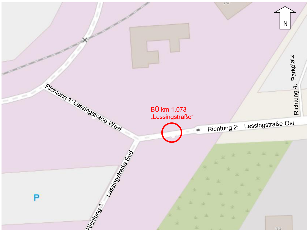
Abbildung 2: Übersicht Einmündungen am BÜ „Lessingstraße“ (Auszug OpenStreetMap 2020)
