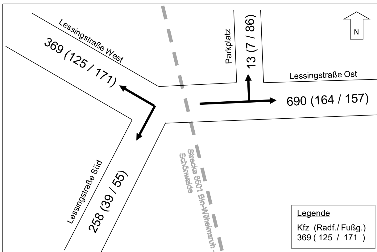
Abbildung 3: Knotenstrombelastung am BÜ km 1,073 „Lessingstraße“
