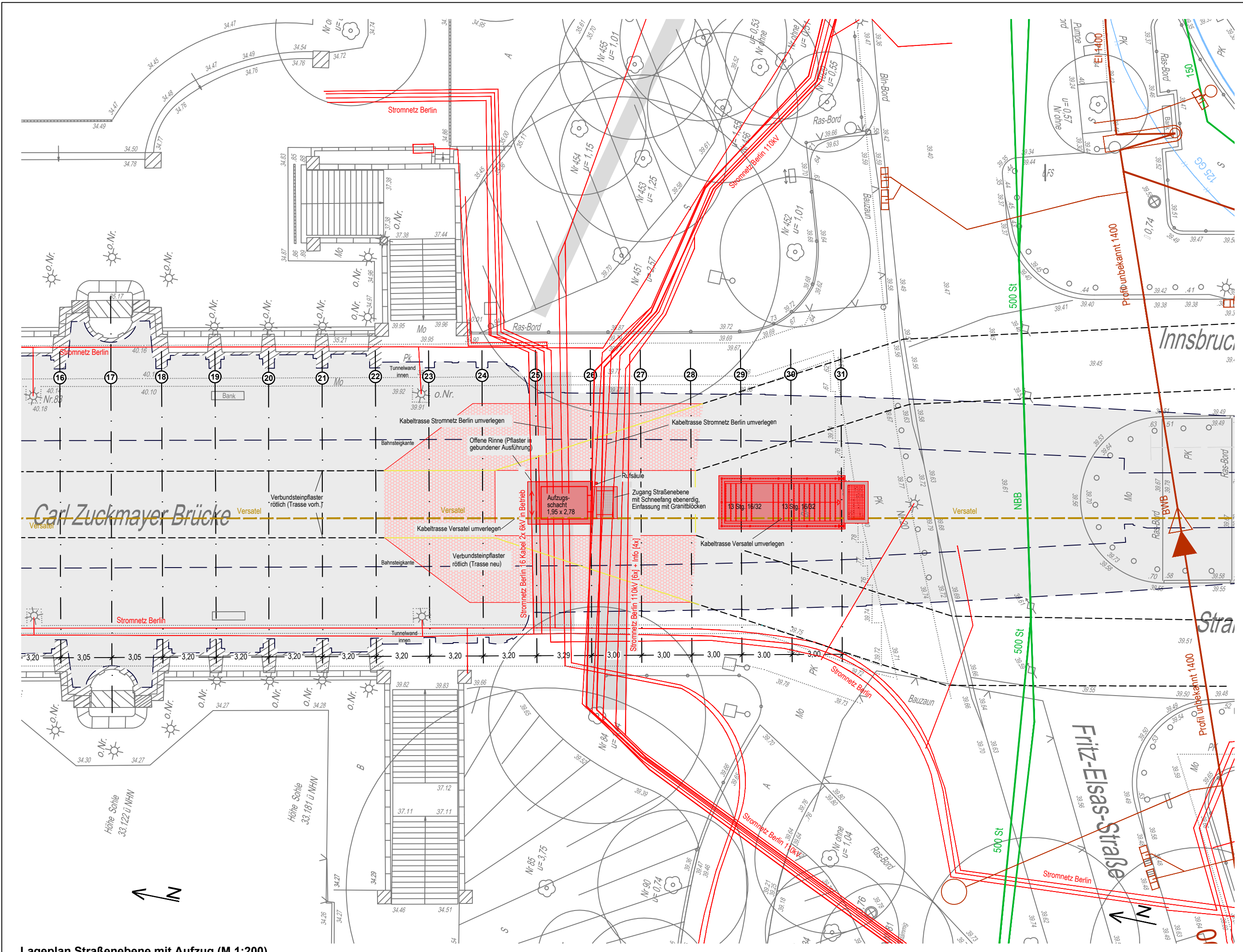
Lageplan Straßenebene mit Aufzug (M 1:200)
