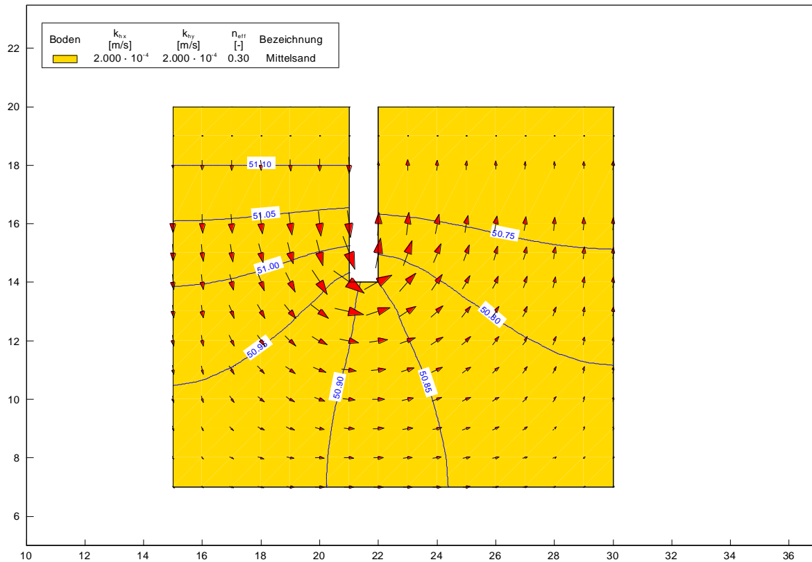
Umströmung Wehr 45 (Draufsicht)
