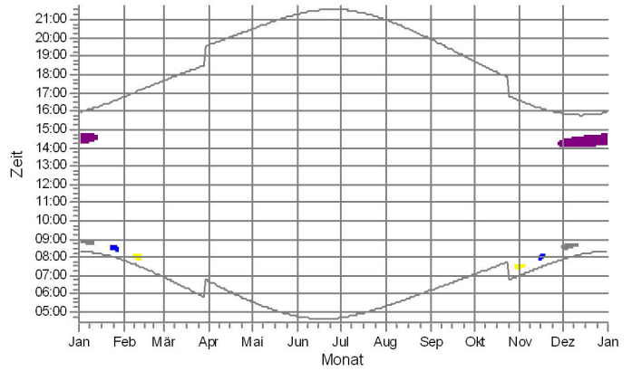
B: IO C Am Schlosspark 1, Mürow, Schatten
