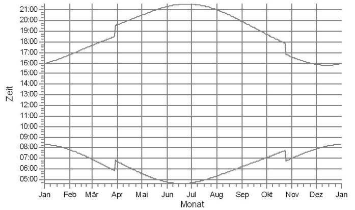
D: IO E Kerkower Straße 2, Dobberzin, Schatten
