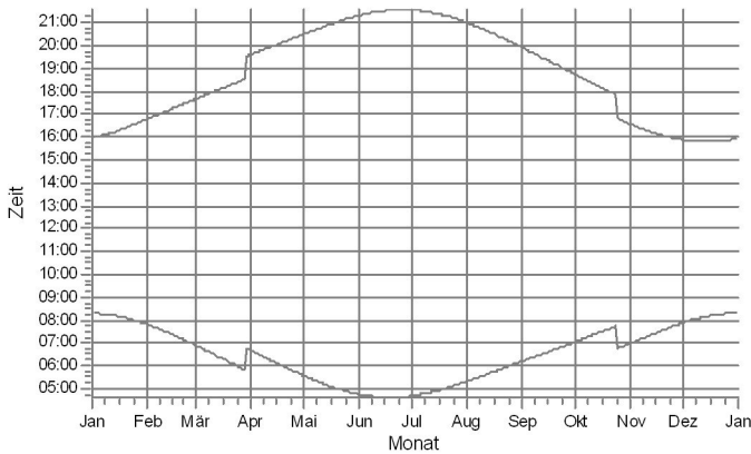
Q: IO S Neuhofer Straße 13, Crussow , Schatten
