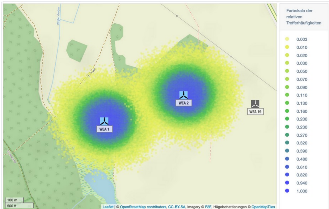
Abbildung A.1.1: Trefferhäufigkeiten von Eisstücken pro Rasterfläche (16m 2 ) und Jahr in der Umgebung der WEA 1 und 2 am Standort Hasenberg (Karte /1.4/).
