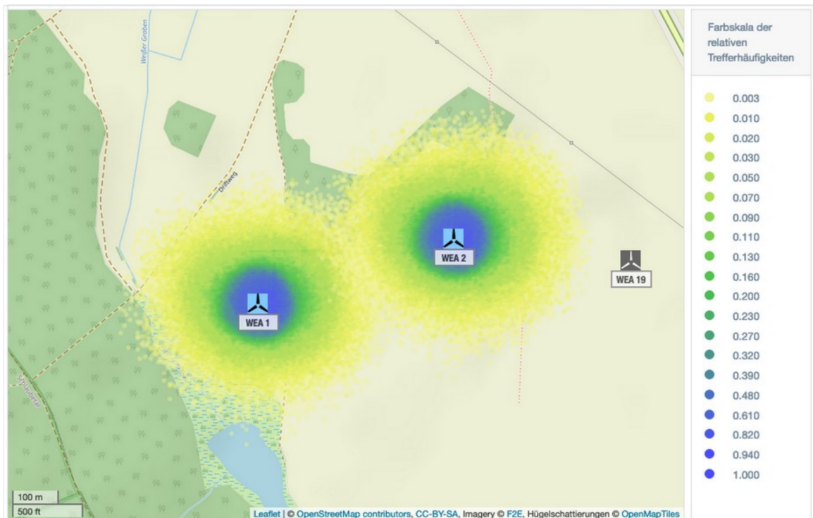
Abbildung B.1.1: Trefferhäufigkeiten von Eisstücken pro Rasterfläche (16m 2 ) und Jahr in der Umgebung der WEA 1 und 2 am Standort Hasenberg (Karte /1.4/).
