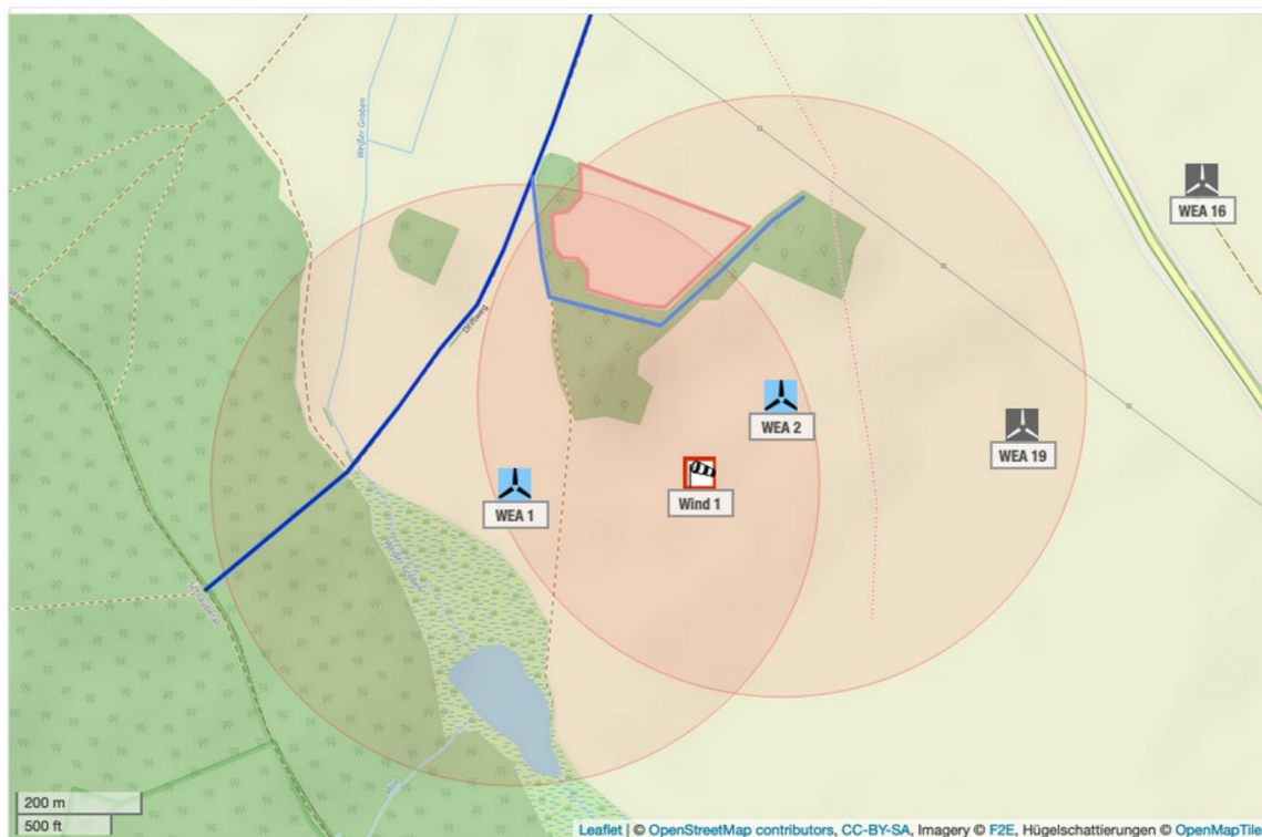
Abbildung 4.3.1: Potentielle Gefährdungsbereiche der WEA 1 und 2 und Schutzobjekte am Standort Hasenberg (Karte /1.4/).
