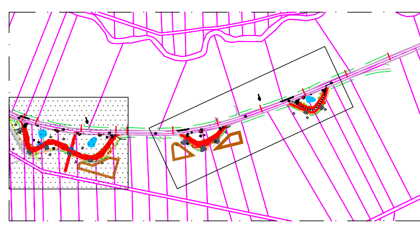
Übersichtsplan o.M.
