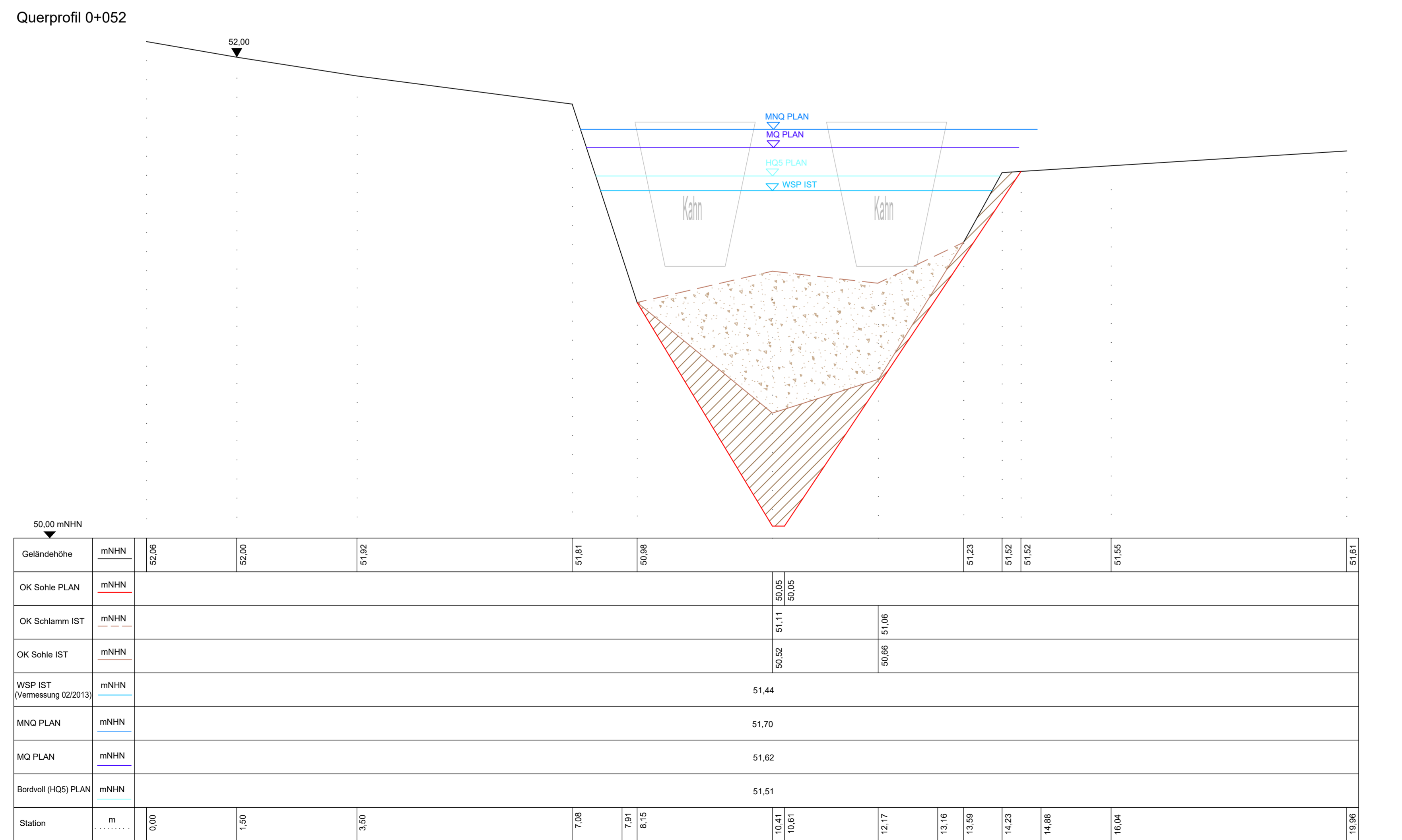
Querprofil 0+052
