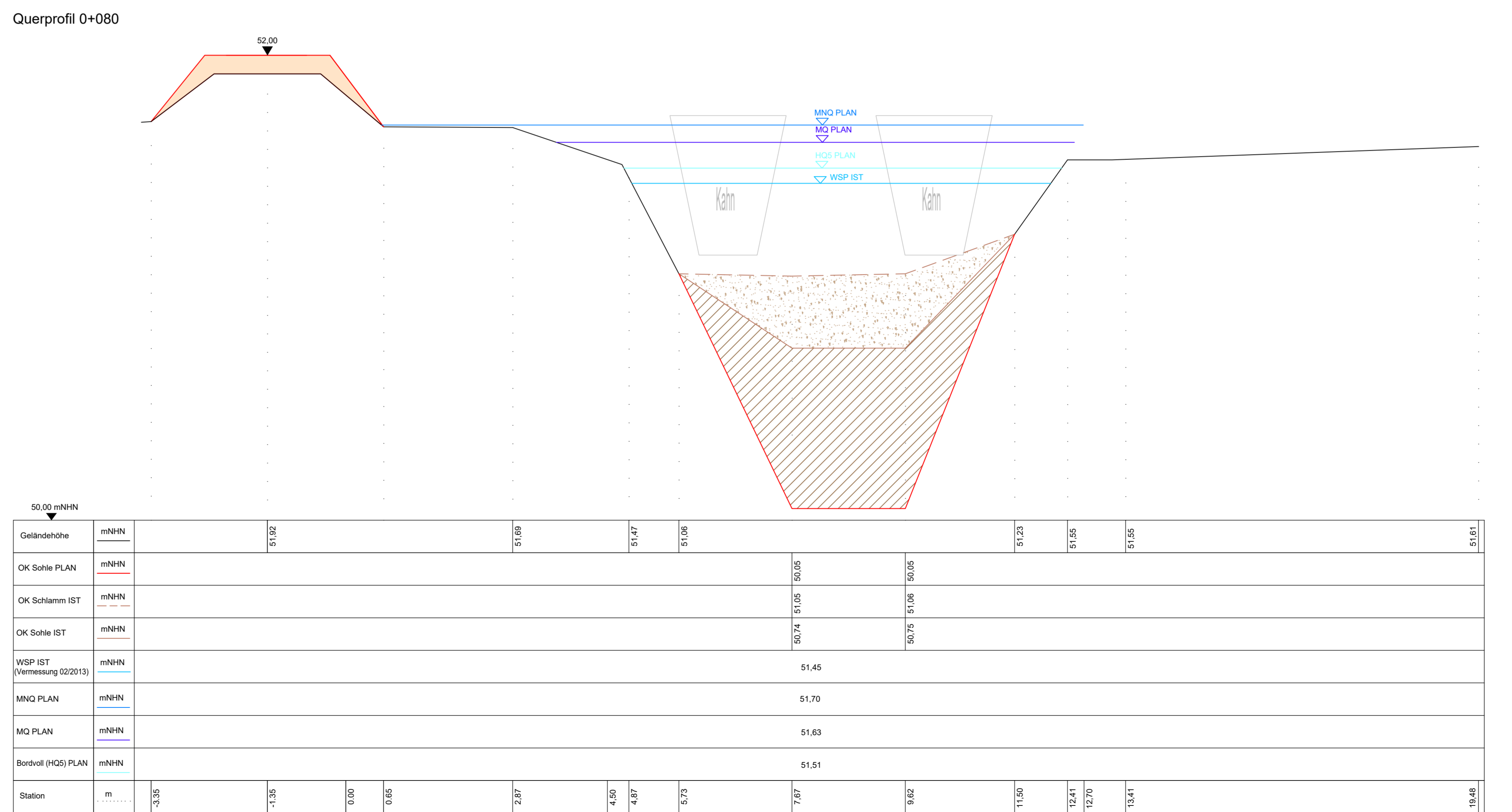
Querprofil 0+080
