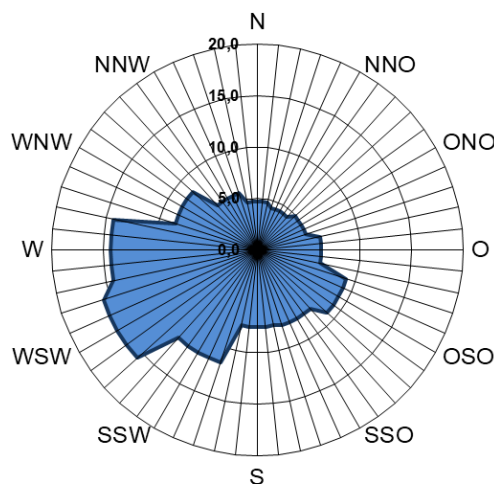
Abbildung 2: Relative Häufigkeit der Windrichtung am Standort Wulkow-Booßen in Prozent (Bezugshöhe 164,0 m ü. Grund) /27/
